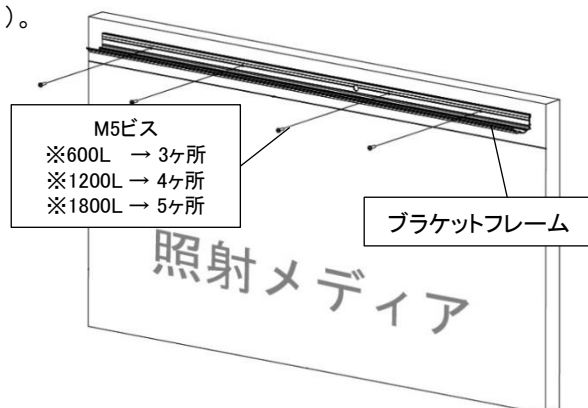
<図2:ブラケットフレームの取付け>
