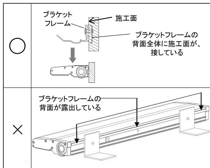
<図3:ブラケットフレーム施工時の注意事項>
