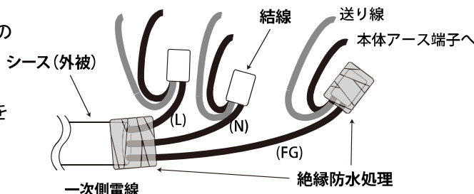
<図7: 配線加工 絶縁テープ処理>
