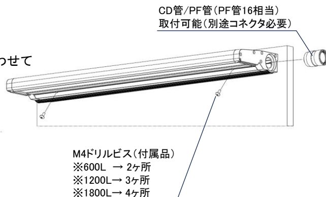
<図6: ボディフレームの組付け>
