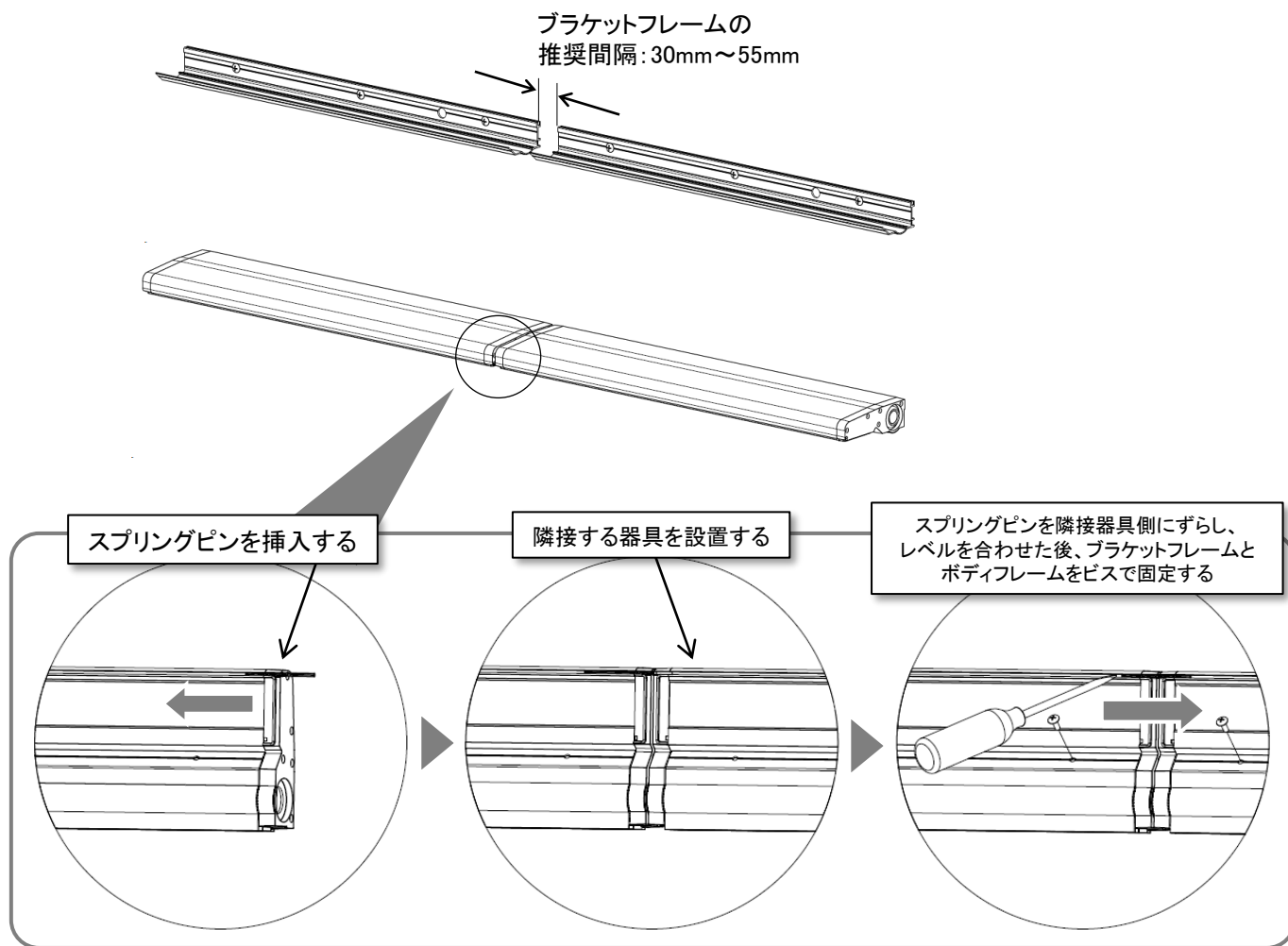
〈図8: 連結設置時の器具のレベル合わせ手順〉
