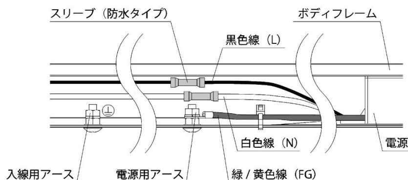
<図4: 一次側電線加工>
