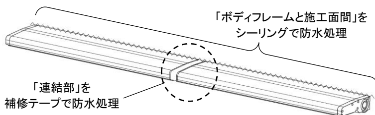
〈図9: 防水処理方法〉
