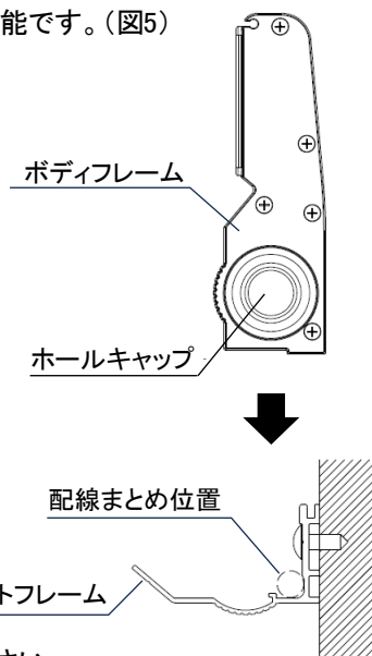
<図5: 配線作業時>
