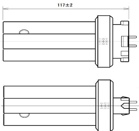
図-1 (単位:mm)
