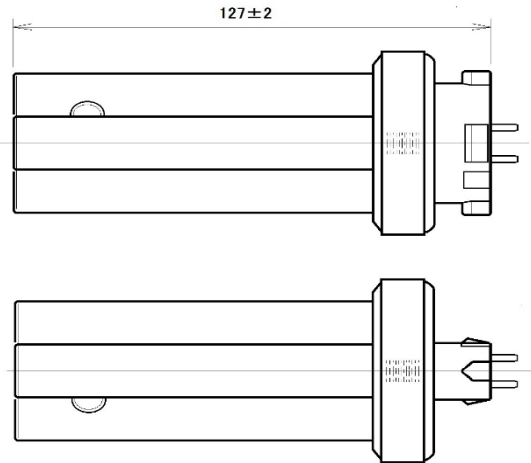
図-1 (単位:mm)
