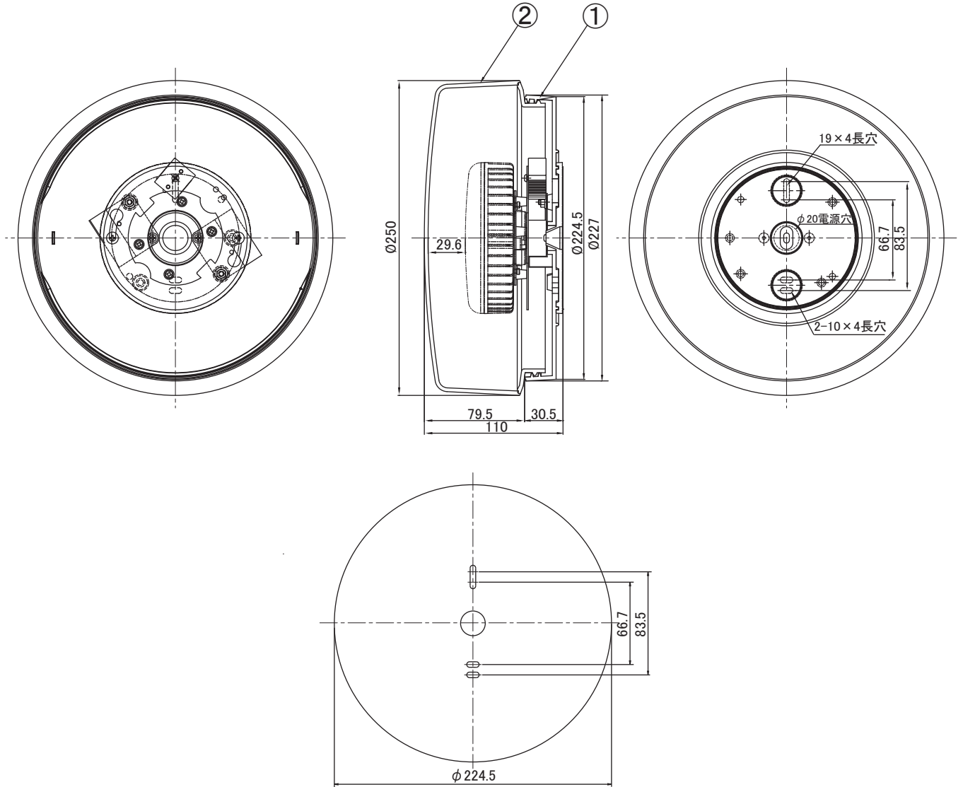
取付寸法図
