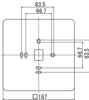
取付寸法図
