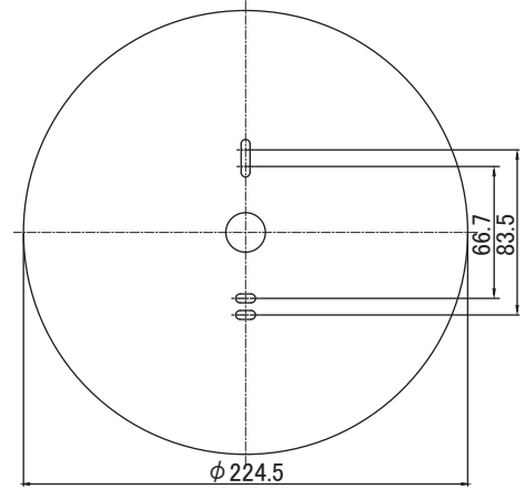
取付寸法図
