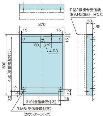
かさ上げボックス BZ5 ☑オーダー
