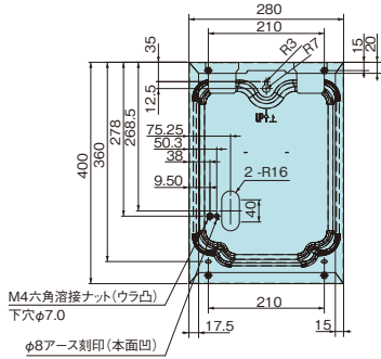
P型2級複合受信機 8回線 BVJ420503H 10回線 BVJ420505H
