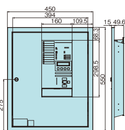
P型2級複合受信機(内器) BZJ11 ☑オーダー
