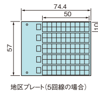
地区プレート(5回線の場合)
