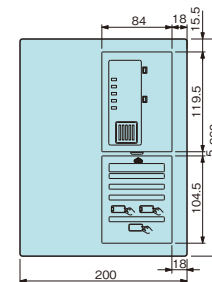
かさ上げボックス BZ5 ☑オーダー
