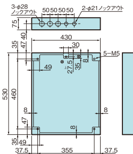
埋込ボックス1型 BVJ8300K
