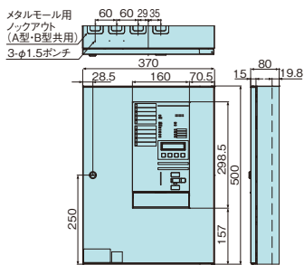
P型2級複合受信機 8回線 BVJ420503H 10回線 BVJ420505H
