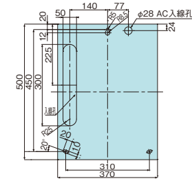
埋込ボックス1型 BVJ8300K
