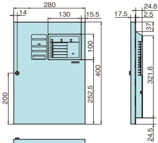
シンプルP-2シリーズ P型2級受信機(ストロングタイプ) 3回線内器 BVJ25231 5回線内器 BVJ25251
