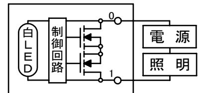
内部回路図
