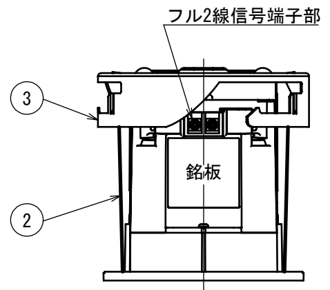
樹脂ケースを外した状態
