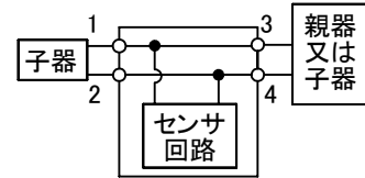
内部回路図
