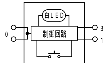
内部回路図
