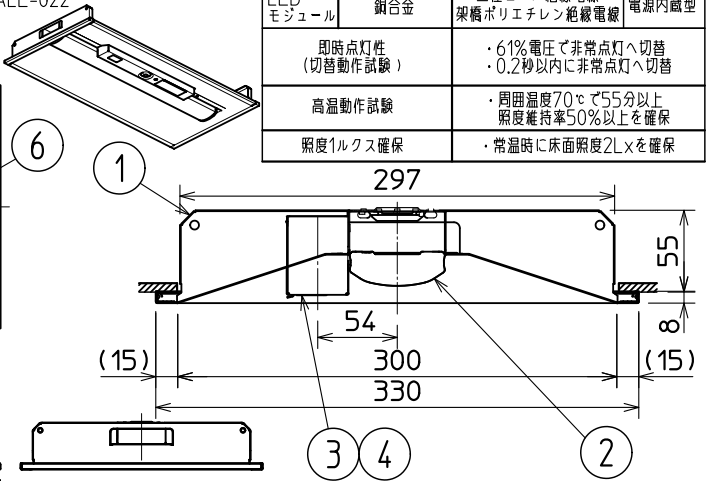
断面詳細図
