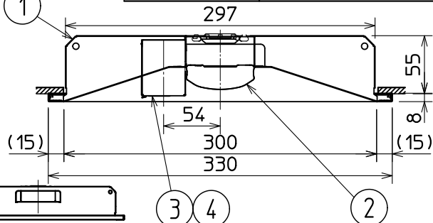
断面詳細図
