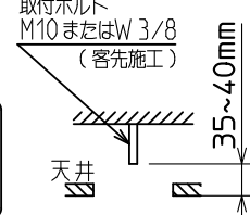
器具取付ボルト長さ
