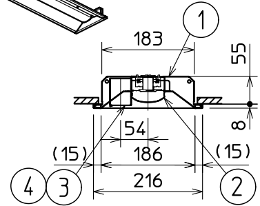
断面詳細図
