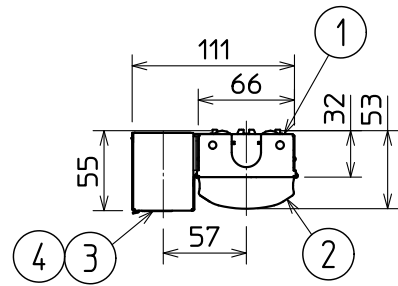
側面詳細図
